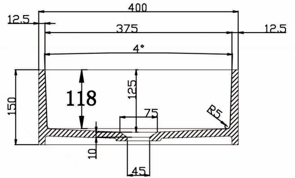
A-A
